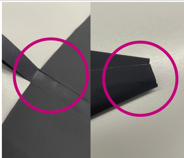
1.Verificare che la saldatura sia allineata correttamente
