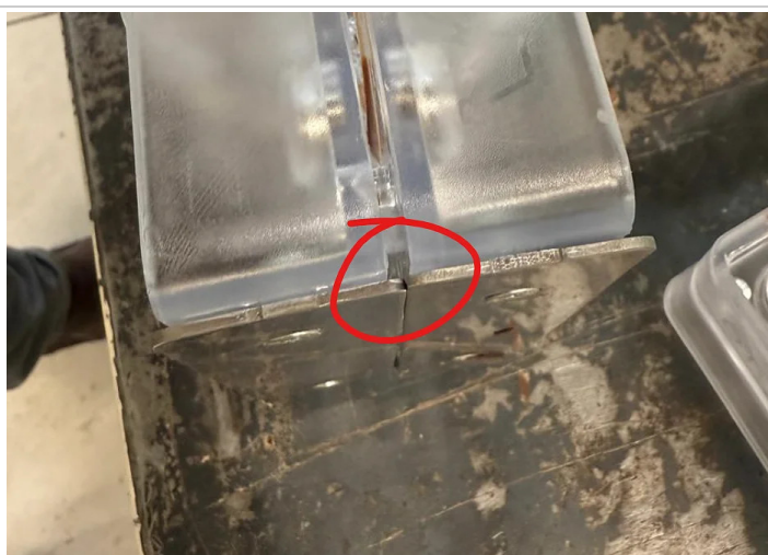
Verificare che le placche siano allineate correttamente allo stampo, altrimenti gli stampi non si chiudono correttamente e il cioccolato esce
